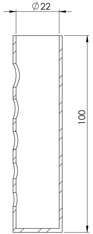
SEÇÃO A-A ESCALA 1 : 1
